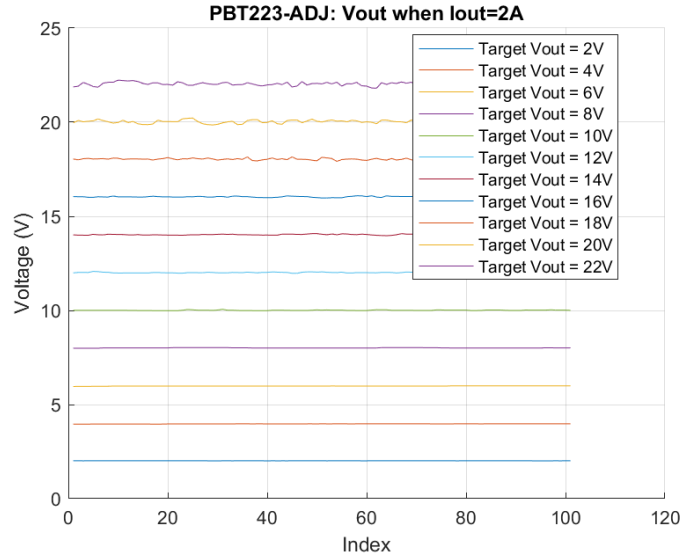
Figure 8 恒电压 CV 模式: Iout=2A
