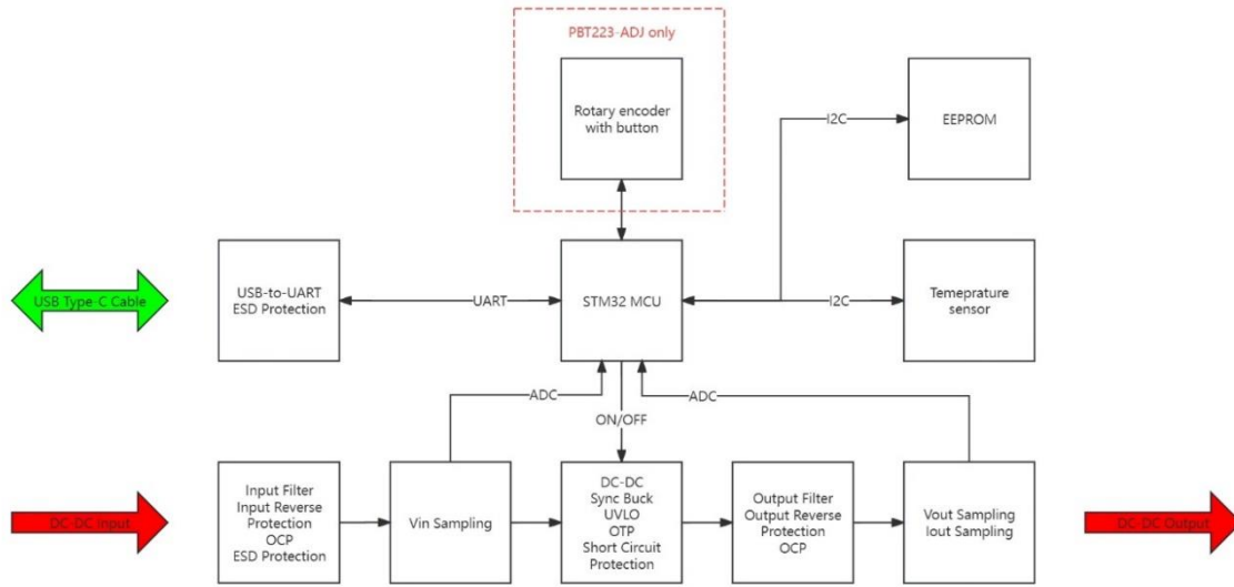
Figure 16 PBT223 功能方框图
