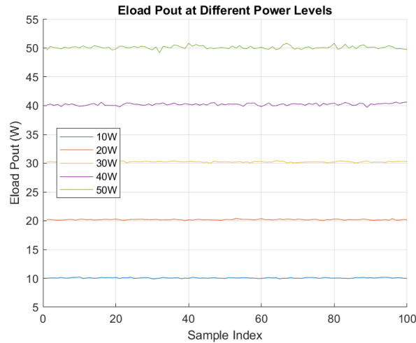
Figure 9 恒功率 CP 模式
